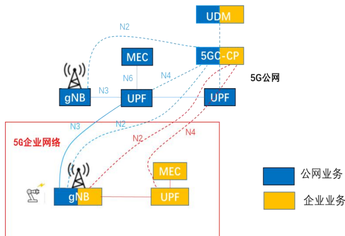
图3 5G混合专网部署方式
