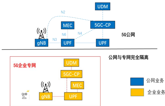
图 5 5G 独立专网部署方式
