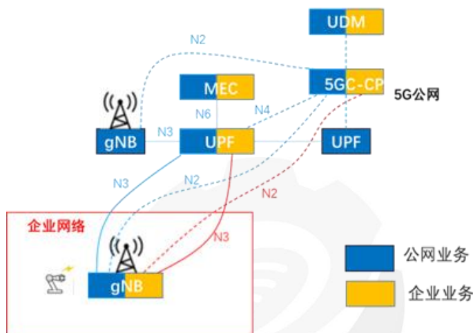
图 4 5G 虚拟专网部署方式
